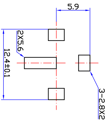
印制线路板推荐开孔尺寸
