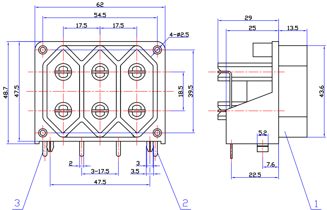
印制线路板推荐开孔尺寸
