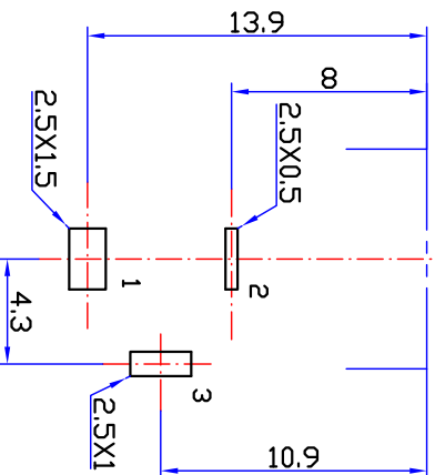
印制线路板推荐开孔尺寸 从下往上插
