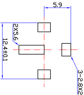
印制电路板推荐开孔尺寸
