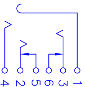
接点示意图
