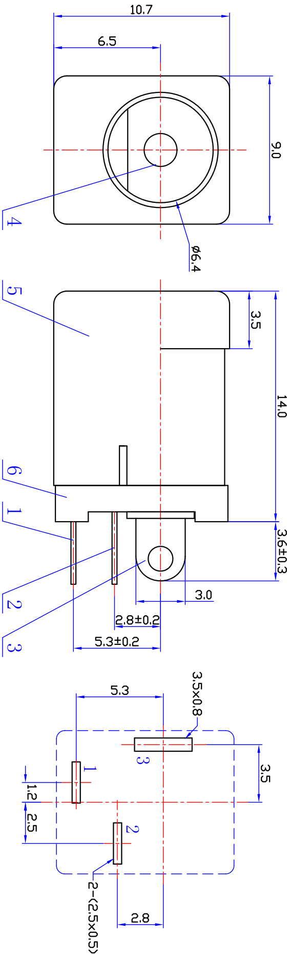
印制线路板推荐开孔尺寸
