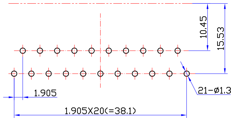
印制电路板推荐开孔尺寸
