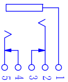
接点示意图
