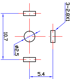
印制线路板推荐开孔尺寸
