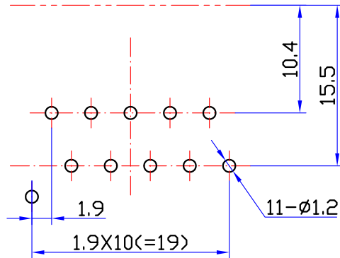
印制线路板推荐开孔尺寸
