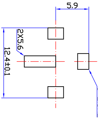
印制线路板推荐开孔尺寸
