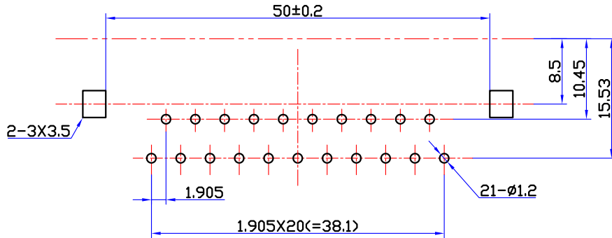
印制线路板推荐开孔尺寸 由下往上插 ⊙
