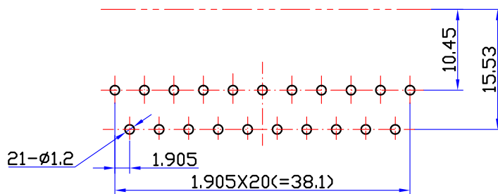
印制线路板推荐开孔尺寸
