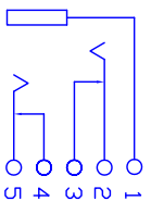
接点示意图
