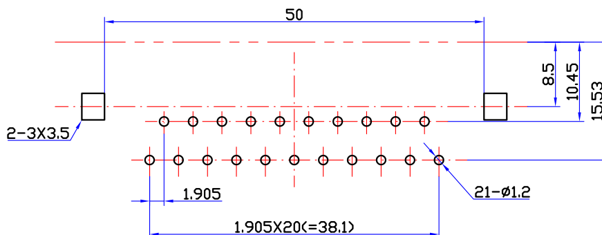
印制电路板推荐开孔尺寸
