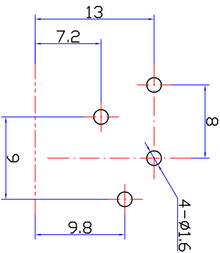
接点示意图
