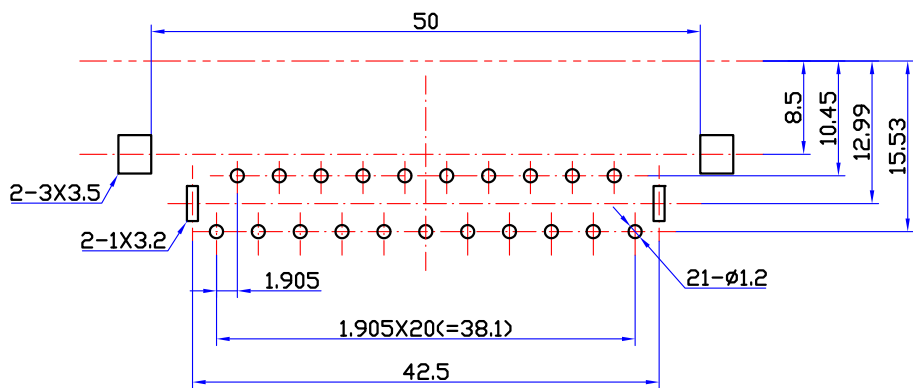
印制电路板推荐开孔尺寸
