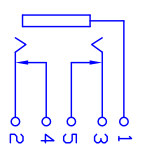
接点示意图
