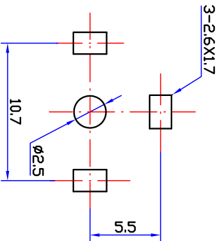
印制线路板推荐开孔尺寸
