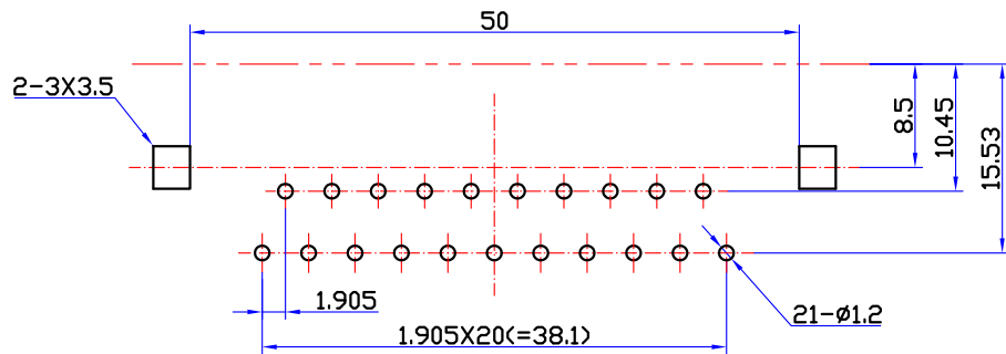
印制电路板推荐开孔尺寸
