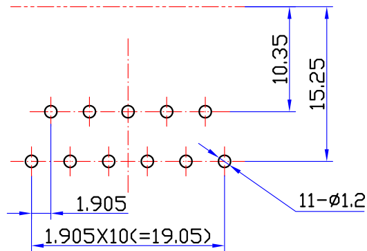
印制线路板推荐开孔尺寸
