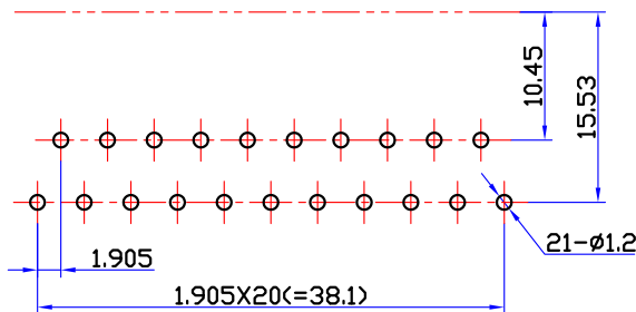
印制电路板推荐开孔尺寸
