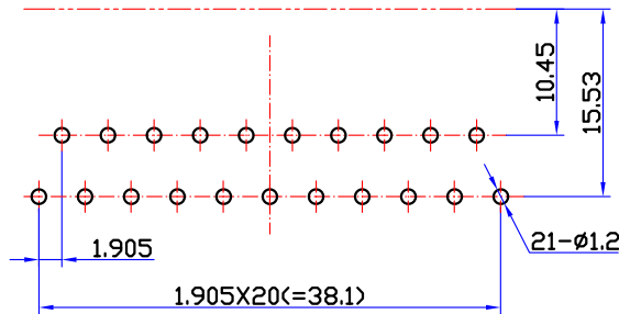
印制线路板推荐开孔尺寸
