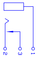
接点示意图
