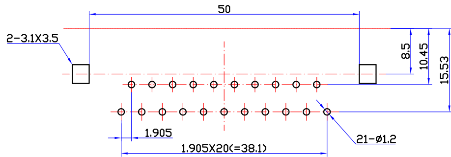
印制线路板推荐开孔尺寸
