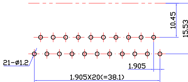
印制电路板推荐开孔尺寸
