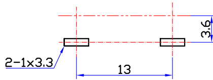
印制电路板推荐开孔尺寸
