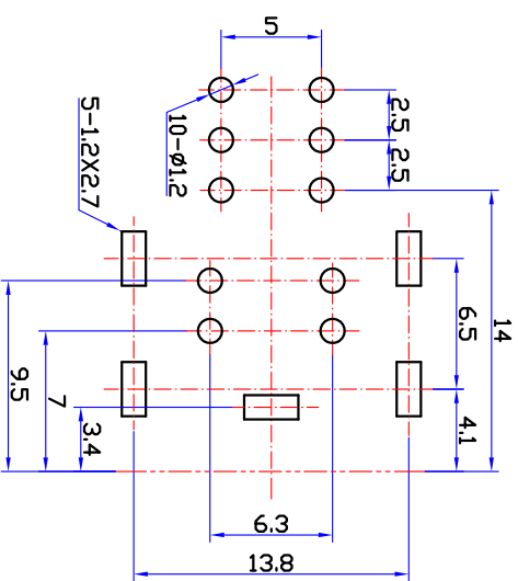
印制线路板推荐开孔尺寸
