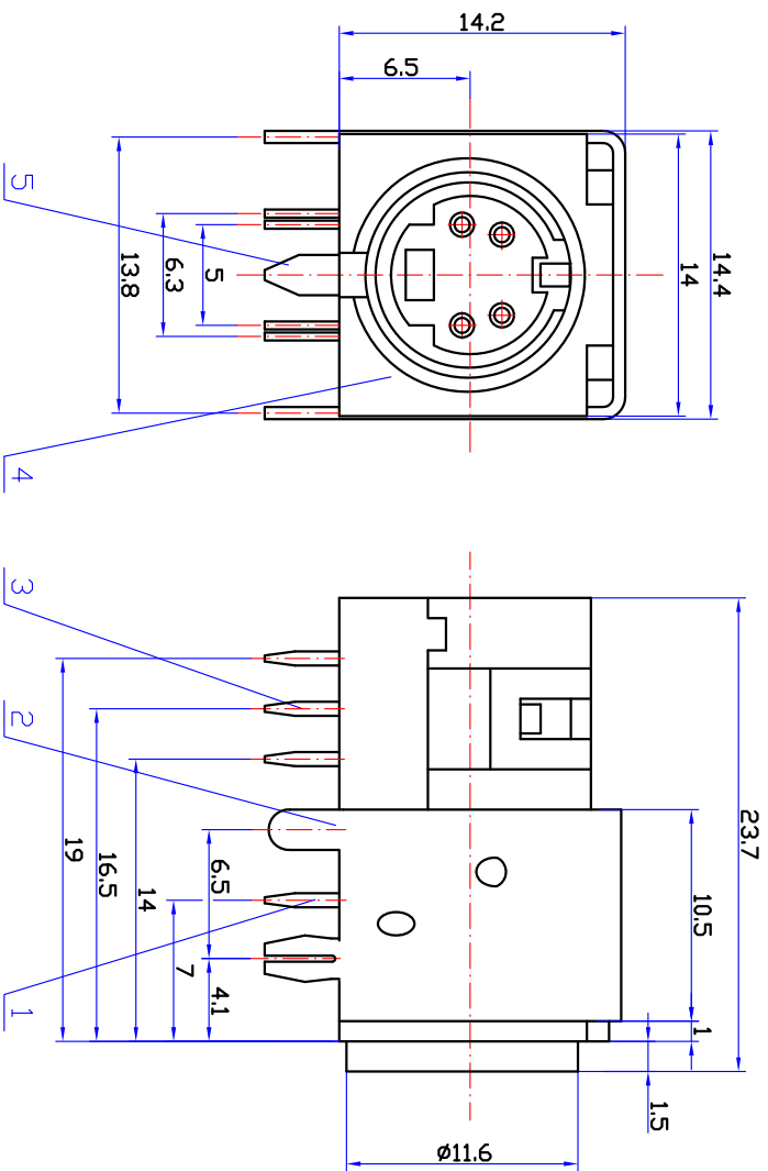
接点示意图
