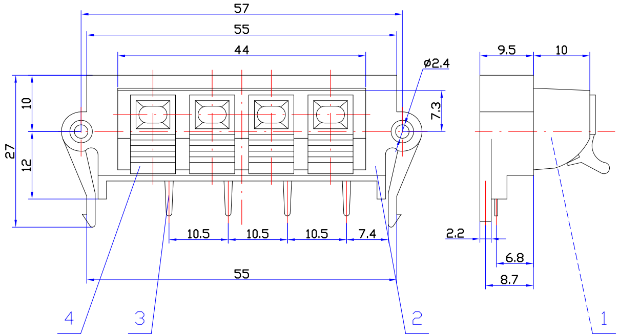
印制线路板推荐开孔尺寸
