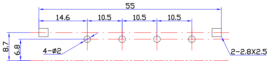
安装板开孔尺寸
