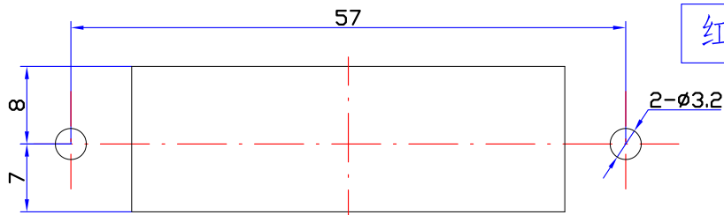
安装板开孔尺寸
