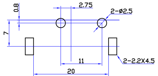
印制线路板推荐开孔尺寸
