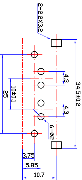
印制线路板推荐开孔尺寸
