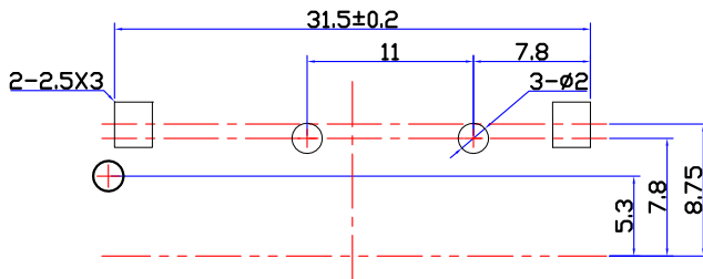
印制线路板推荐开孔尺寸
