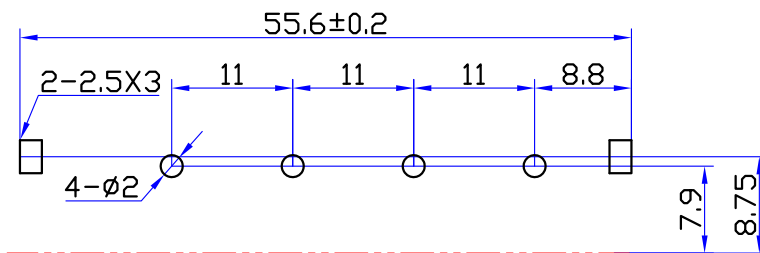
印制线路板推荐开孔尺寸
