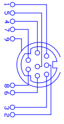
接点示意图
