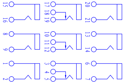
接点示意图
