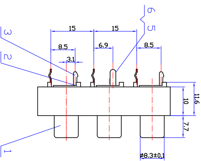
接点示意图
