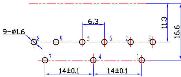
印制线路板推荐开孔尺寸 由下往上插
