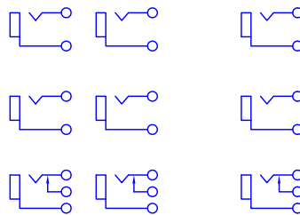
接点示意图
