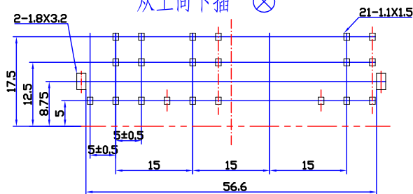
印制线路板推荐开孔尺寸
