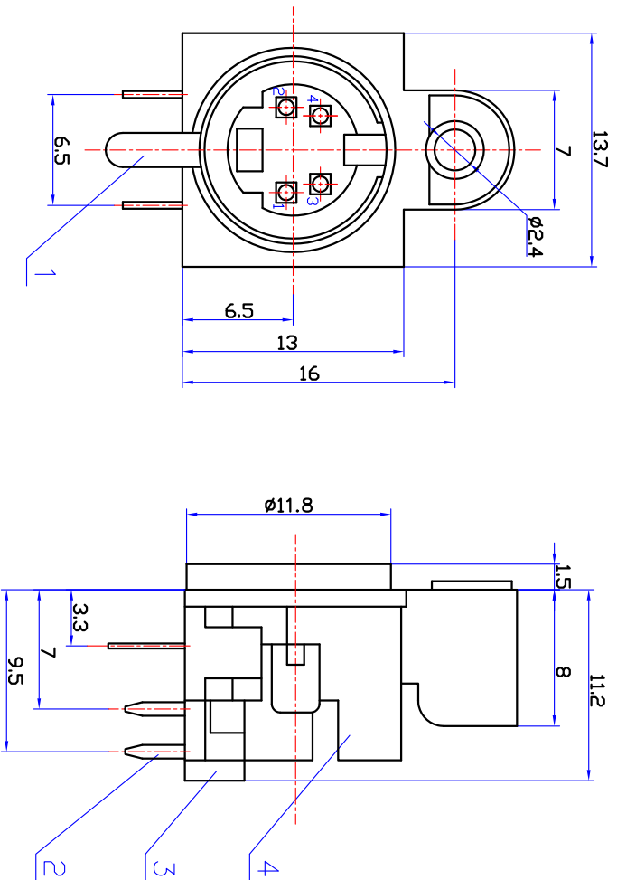
接点示意图
