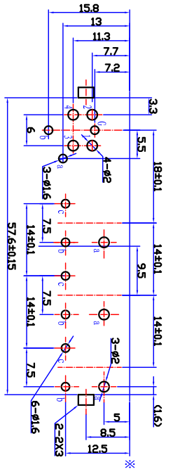
印制电路板推荐开孔尺寸 由下向上插
