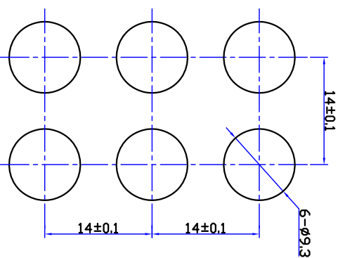
安装板开孔尺寸
