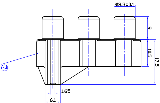
接点示意图
