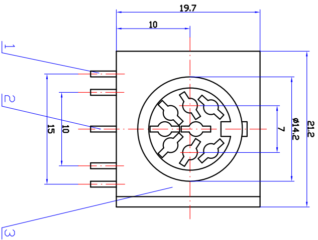
接点示意图
