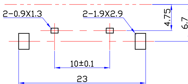
印制电路板推荐开孔尺寸 从下向上插
