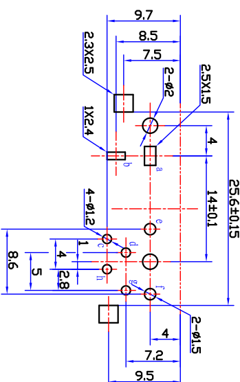
印刷线路板推荐开孔尺寸 由向上插
