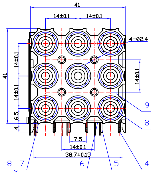
印制电路板推荐开孔尺寸 由下向上插
