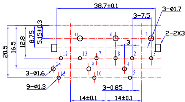
印制电路板推荐开孔尺寸 由下向上插
