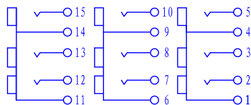
接点示意图
