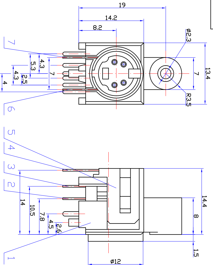
接点示意图
