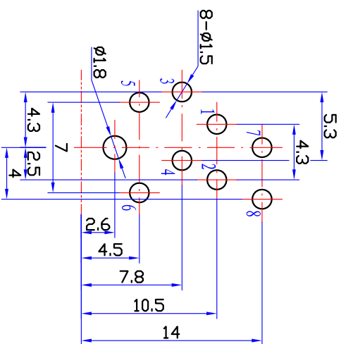
印制线路板推荐开孔尺寸
