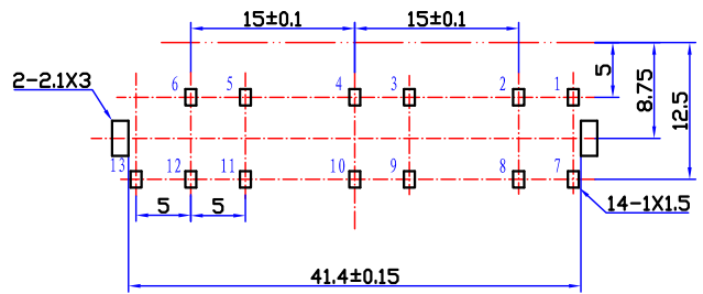
印制线路板推荐开孔尺寸
