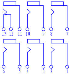
接点示意图
