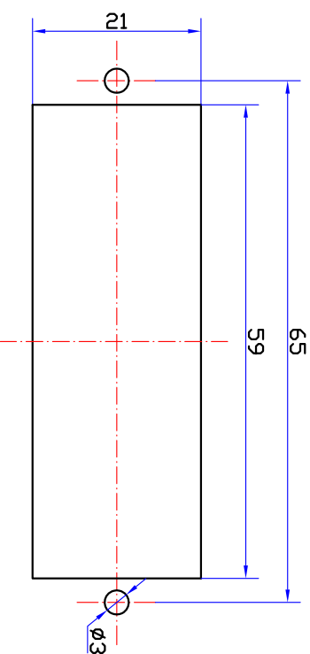
安装板推荐开孔尺寸
