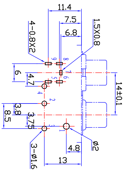
印制线路板推荐开孔尺寸 由向下上插
