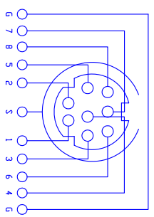
接点示意图
