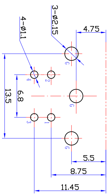
印制线路板推荐开孔尺寸 从下往上插
