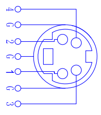
接点示意图
